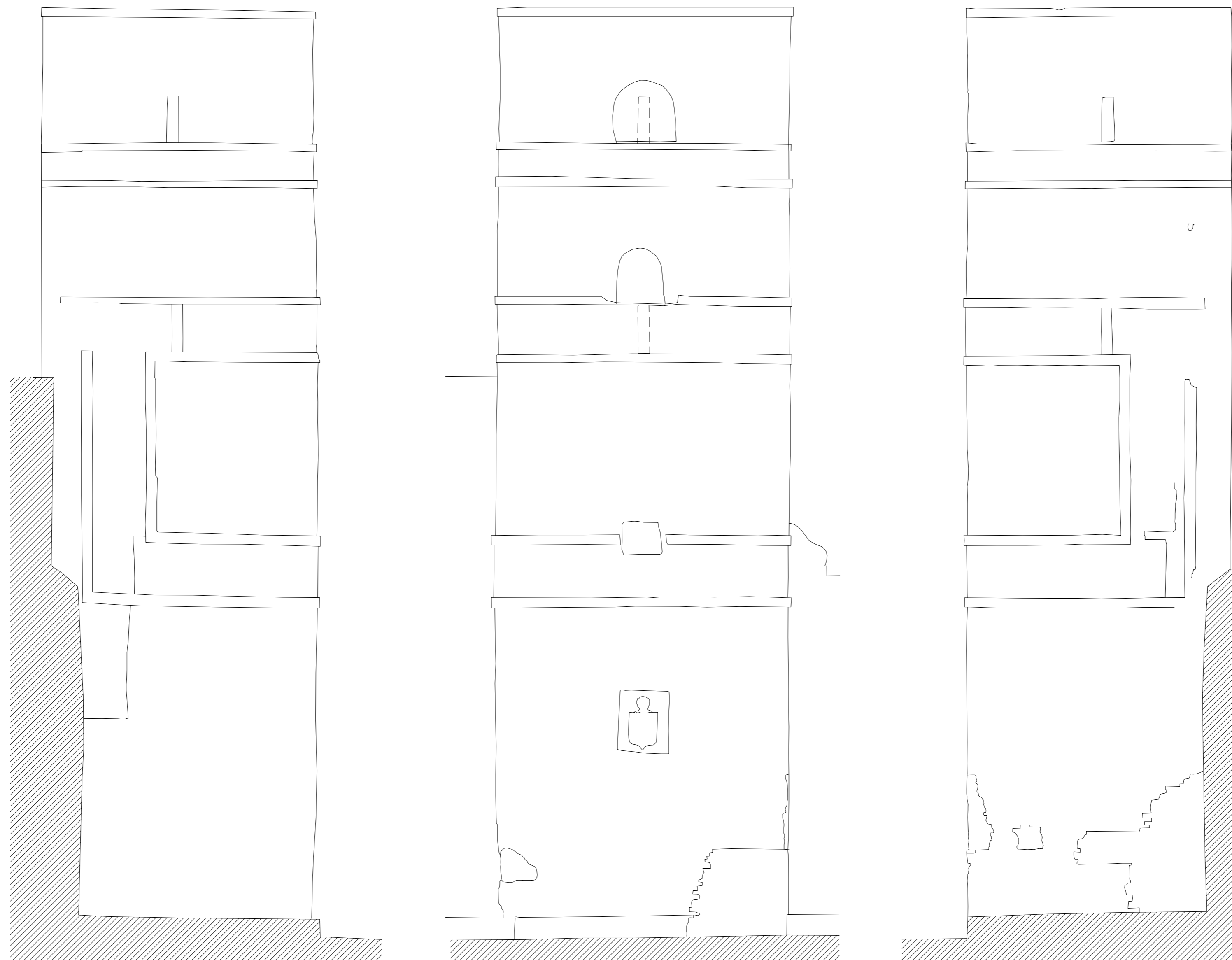
ALZADOS DE LA TORRE EXISTENTE ENTRE LA PLAZA DE ALFARO Y LA CALLE DE NICOLAS ANTONIO
