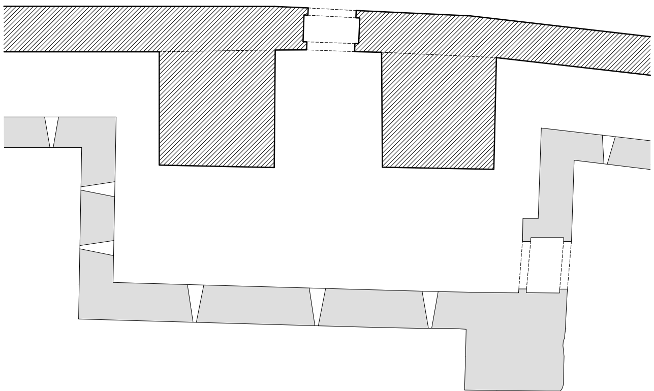
PLANTA HIPOTESIS
